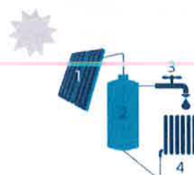
1 Zonnecollector | 2 Opslagvat zonneboiler | 3 Sanitair warm water | 4 Afgifte-energie voor ruimteverwarming (optioneel)
